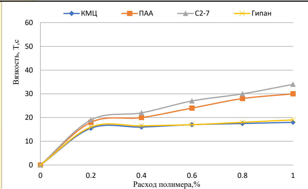
Рис. 1. Влияние концентрации полимеров на условную вязкость минерализованных (NaCl 5 %) 5 % суспензий НЦБ: 1) КМЦ; 2) ПАА; 3) С2-7; 4) Гипан.
