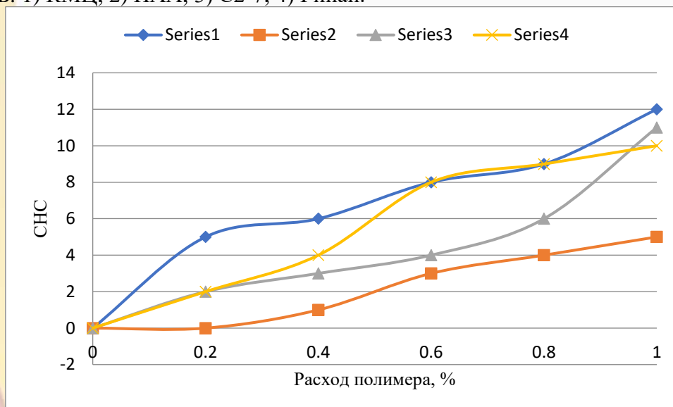
Рис. 2. Влияние концентрации полимеров на СНС минерализованных (NaCl 5 %) 5 % суспензий НЦБ: 1) КМЦ; 2) ПАА; 3) С2-7; 4) Гипан.
